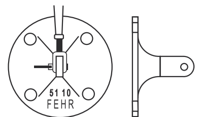
Kuva 2.3: Seinäkiinnike alumiini
